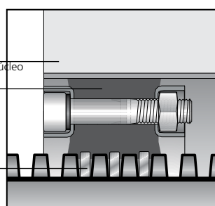
Vista de detalle Clip de anillo/sello
