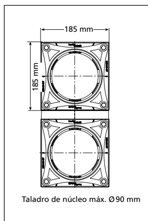
Brida de aluminio HSI90 DF
