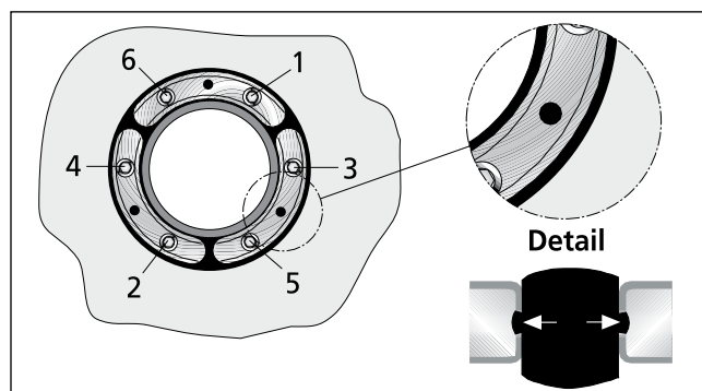
Vista detallada – HSD
