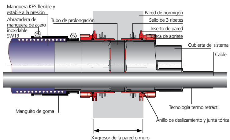
Canalización de estaciones: Cable de baja tensión sellado con HSI150 D1x80 WS
