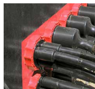
Canalización de estaciones: Cable de baja tensión sellado con HSI90 D1x75 WS and HSI90 D3x32 WS
