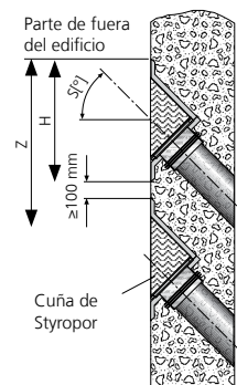
2x HSI90 1xZ K S45°/X Empaquetadura inclinada sencilla
