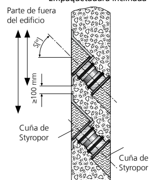
2x HSI90 1xZ- K2 S45°/X Empaquetadura inclinada doble
