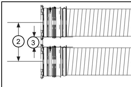
2 Rozstaw otworów w osi 250 mm
