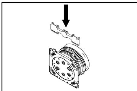
1 Schalungsabstand
