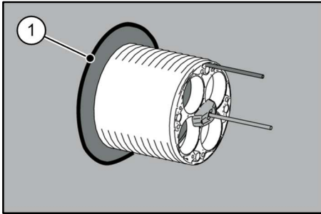
1 Austritt Butylband
