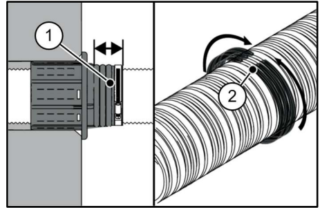
1 Bereich Adapterring/Spannband
