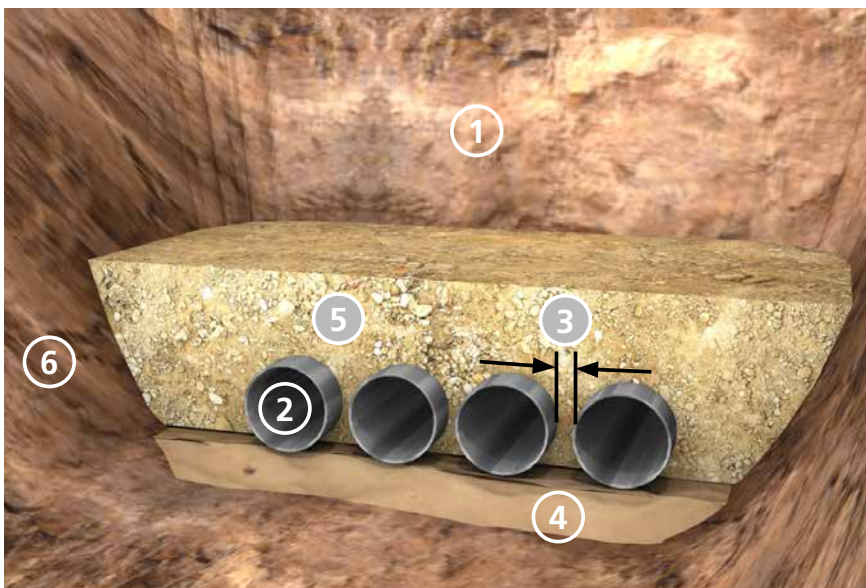
Einlagiges Hateflex-Schlauchsystem
