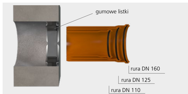
Uniwersalne wkłady uszczelniające HSD200 SSG 1x110/125/135/160 b40 umożliwiają uszczelnianie standardowych rur kanalizacyjnych
