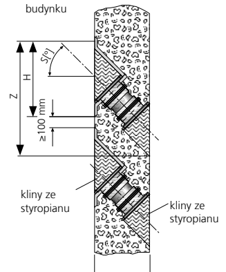
2x HSI150-1xZ-K2S45°/X dwustronny przepust kątowy do zabetonowania
