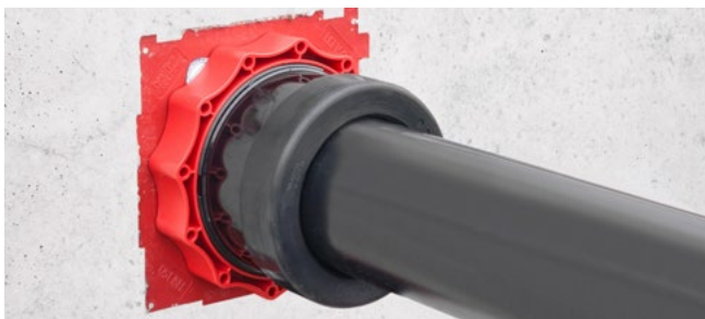
uszczelnienie gładkiej rury osłonowej \varnothing 125 pokrywą systemową z mufą wtykową HSI150 D 1x125 GSM
