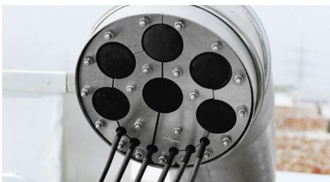
przepust SHD 200 z gumowym wkładem uszczelniającym SKD
