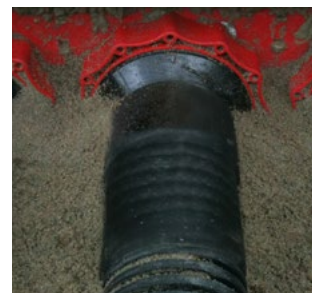
uszczelnienie rur karbowanych pokrywą systemową z opaskami zimnokurczliwymi HSI150 D1x110 KS WR
