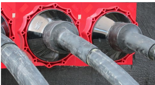
stacja kontenerowa: kable średniego napięcia uszczelnione za pomocą HSI150 D1x80 WS
