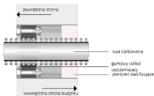
przekrój poprzeczny pozycjonowanie wkładu w otworze
