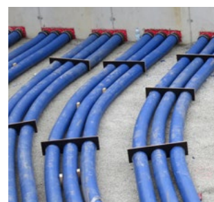
system prowadzenia i osłony kabli KES z użyciem elastycznej rury osłonowej Hateflex
