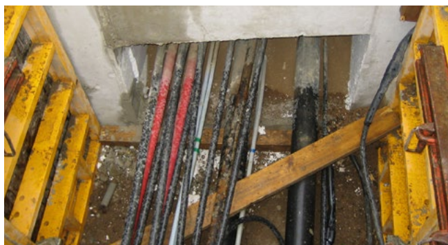
ukośne ułożenie rur i przewodów w otworze
