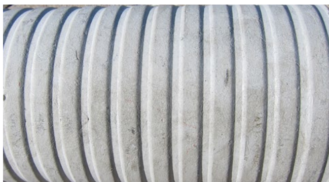
obwodowe rowkowanie zewnętrzne dla lepszego połączenia z budowlą
