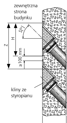
2x HSI150-1xZ-KS45°/X jednostronny przepust kątowy do zabetonowania
