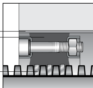
vue détaillée anneau clipsable/étanchéité
