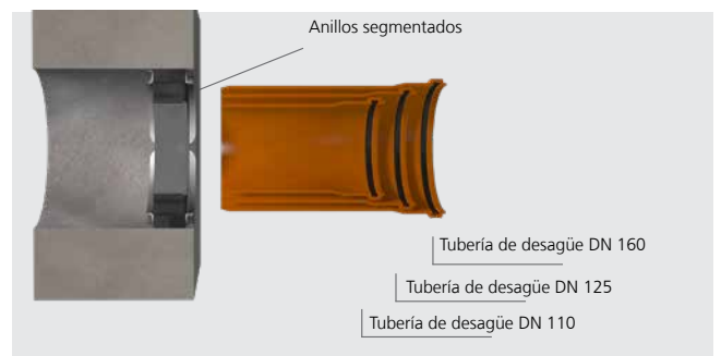
Con el sello redondo universal HSD200 SSG 1x110/125/135/160 b40 se pueden sellar tuberías estándar de \varnothing_e 110, 125 y 160.
