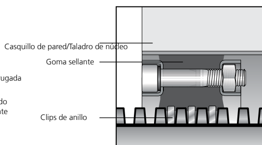
Vista de detalle Clip de anillo/sello
