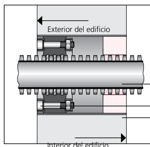
Dibujo en sección Colocación en la abertura
