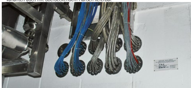
HRD150 G b30 mit Mehrfachbelegung
