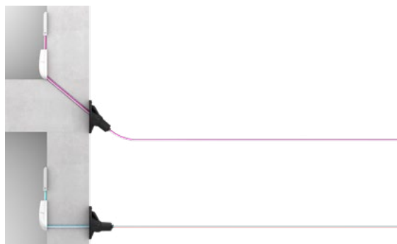
GFH20 PRO - Schräger und waagrecht Einbau
