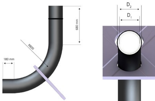
D1: Rohrbogen Øi, D2: Rohrbogen Øa
