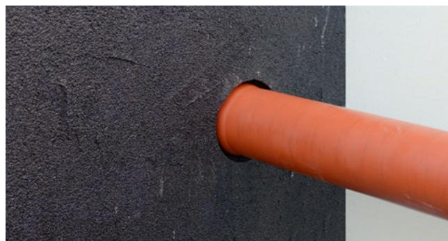
Praxisbild UDM/UDME eingebaut mit angearbeiteter PMBC-Beschichtung und angeschloss-nem KG-Rohr
