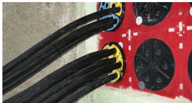
Abdichtung von Kabeln für Straßenbeleuchtung mit SEGMENTO
