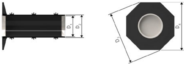
D1: Futterrohr Ø1, D2: Futterrohr Øa, D3: Flansch Kantenmaß, D4: Flansch Flächenmaß
