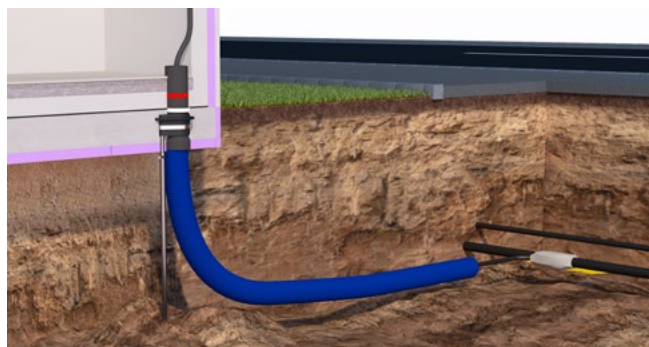
Eingebaute Einsparten-Gebäudeeinführung ESG100 FUBO EBT mit werkseitig verbundenem Leerrohrsystem Hateflex14110, eingebauter Ringraumdichtung HRK100 SSG 1x18-65 und der Sparte Elektro
