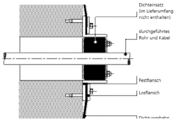
Schnitt - Einbau
