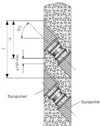
2x HSI150 1xZ K2 S45°/X Doppel-Schrägdichtpackung
