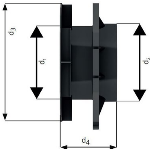
D1: Futterrohr \varnothing_i , D2: Futterrohr \varnothing_a , D3: Flansch Flächenmaß, D4: Mindestwandstärke
