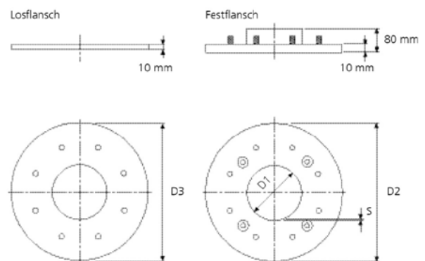
Bemaßung
