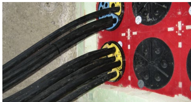
Abdichtung von Kabeln für Straßenbeleuchtung mit SEGMENTO
