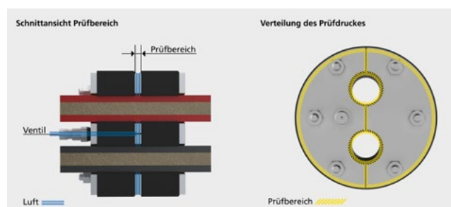
HRD150 PV G in Kernbohrung
