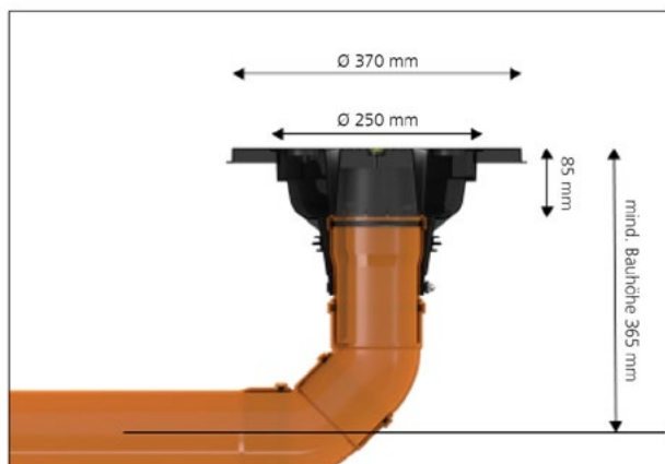
Vermaßung Anschlussstrichter AT110
