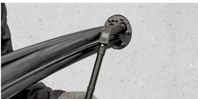
HRD150 PV G in Kernbohrung
