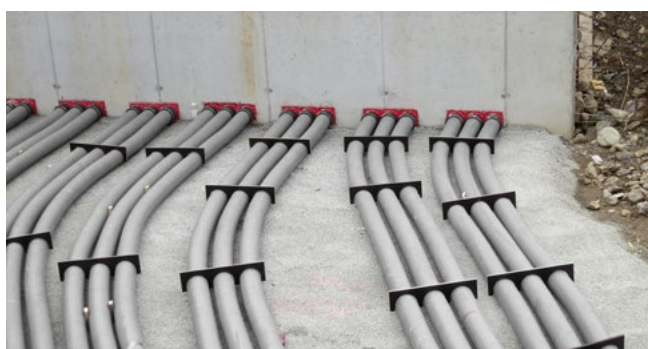
KES MA150 D und Spiralschlauch Hatflex14150
