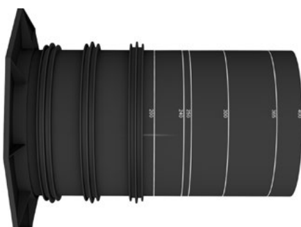
D1: Futterrohr Øi, D2: Futterrohr Øa, D3: Flansch Kantenmaß, D4: Flansch Flächenmaß
