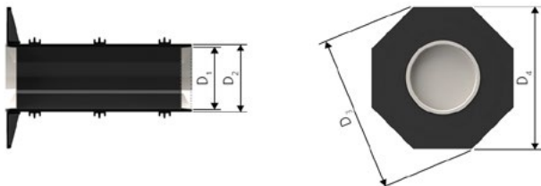
D1: Futterrohr Øi, D2: Futterrohr Øa, D3: Flansch Kantenmaß, D4: Flansch Flächenmaß
