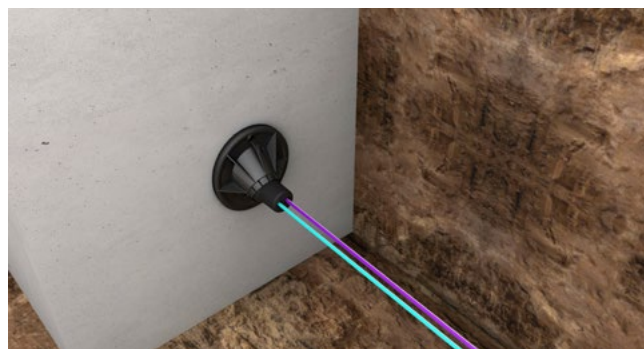
Einbaugrafik - GFH30
