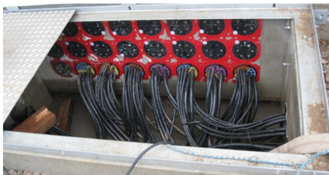
HSI150 - Dichtpackungen bestückt mit SEGMENTO-Abdichtung von Steuerleitungen in einem Schalttafel
