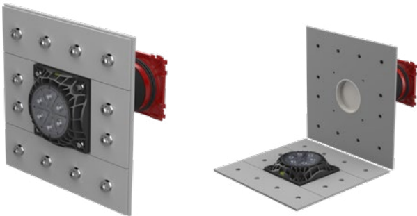
Doppel-Dichtpackung HSI150 1x1 FLFE/X (Vorderansicht). Fest- / Losflansch zum Einbetonieren mit Dichtflansch zum Anschluss von Systemabdichtungen.
