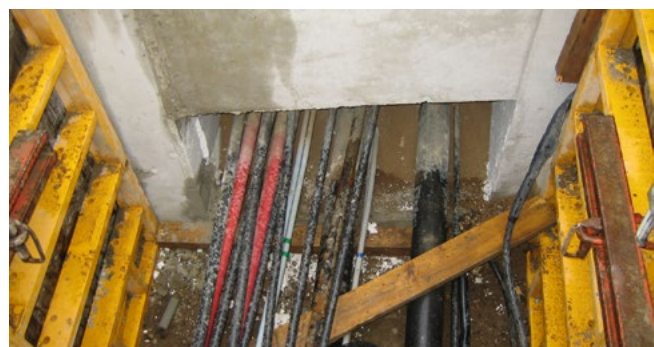
Bauseitig vorhandene rechteckige Aussparung - muss nachträglich abgedichtet werden
