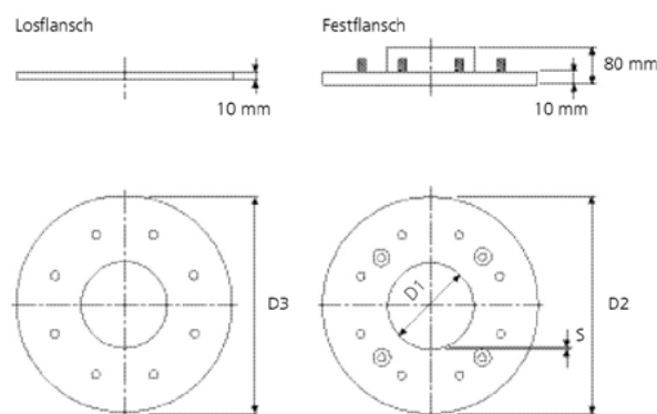
Bemaßung
