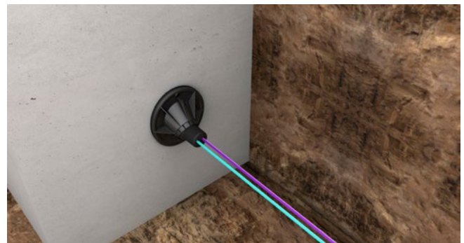
Einbaugrafik - GFH30
