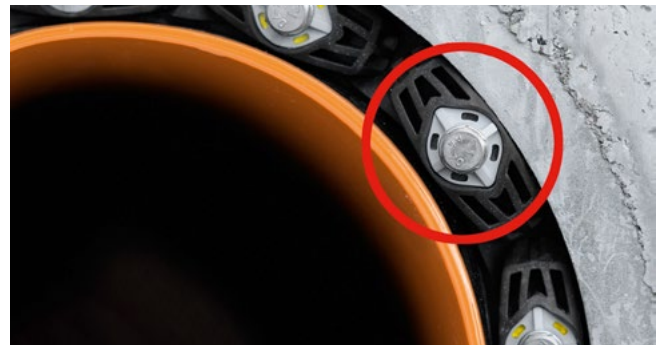
GKD mit einem nicht angezogenen Segment - Montagefehler sofort erkannt
