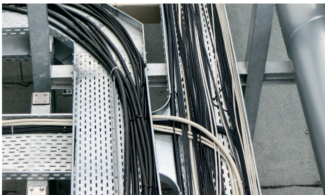
Draufsicht fachgerecht montierte Blindabdichtungen zum Verschluss der Dachtraverse
