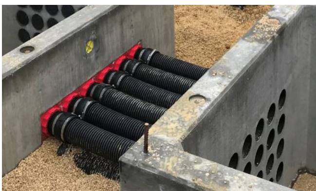
De kabelschachten zijn aan elkaar gekoppeld via in de fabriek gemonteerde HSI 150-afdichtpakkingen, mantelbuizen en onze systeemdeksels HSI 150 – M168 WR.
